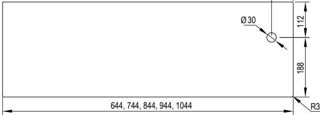
Panel ochronny środkowy z otworami pod zamek oszczędnościowy
