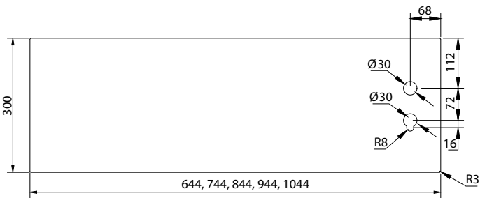
Panel ochronny środkowy z otworami pod zamek wc/klucz/wkładkę
