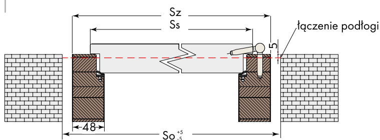
Ościeznica z stałą
