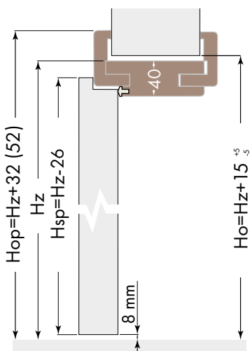
Ościeznica z panelem
