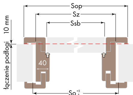
Ościeznica regulowana opaski 60 (80)mm skrzydło bezprzylgowe
