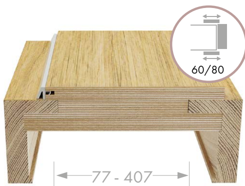
Ościeżnica regulowana PODSTAWOWA
