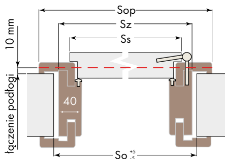
Ościeznica regulowana opaski 60 (80)mm skrzydło przylgowe
