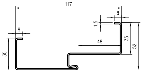
Profil ościeżnicy
