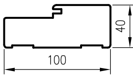
Profil OPB
