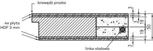
Skrzydło drzwiowe antywłamaniowe-przeciwpożarowe Forca B
