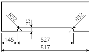
PODCIĘCIE WENTYLACYJNE LUMEN/LUMEN LOFT
