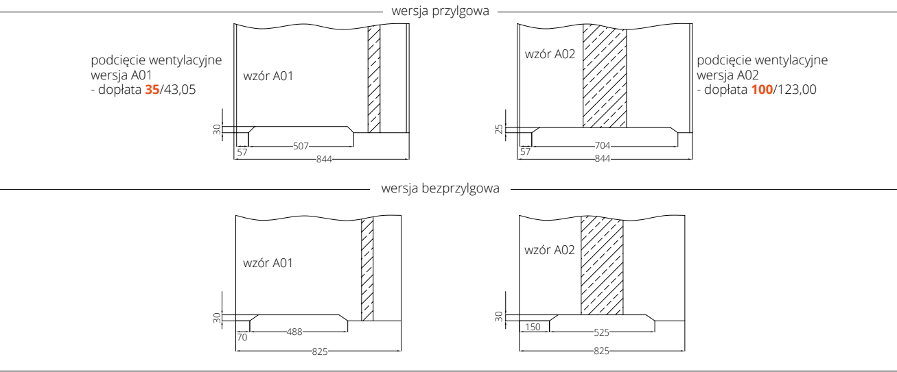
PODCIĘCIE WENTYLACYJNE LUMEN/LUMEN LOFT
