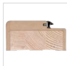
OŚCIEŻNICA STAŁA drewniana w RC2 lub wzmocniona w RC3
