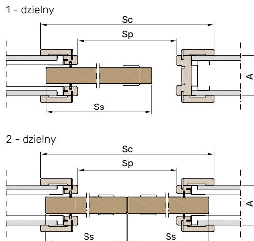
System wewnątrzścienny
