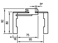
Przekrój ORB 075
